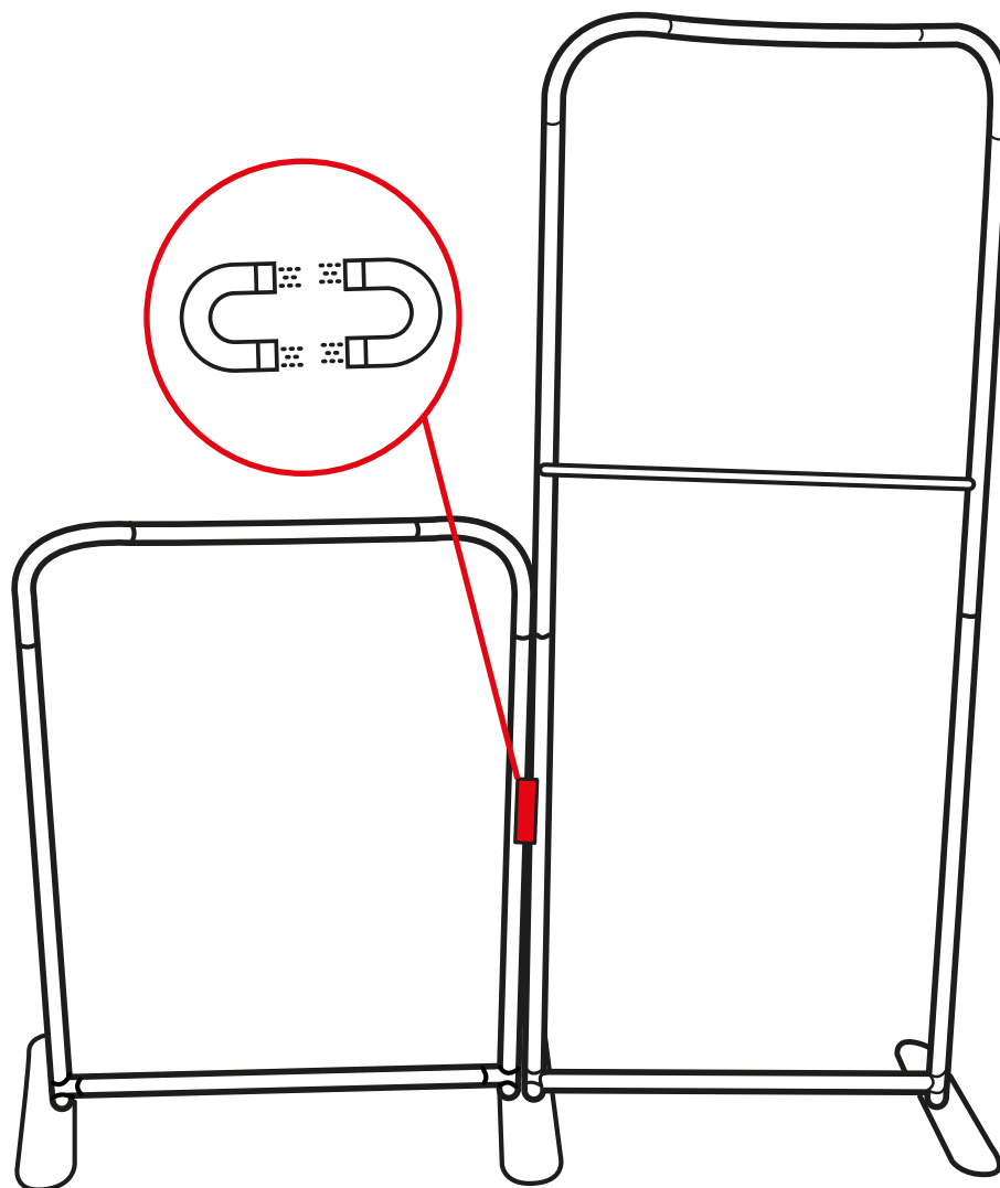
Рамка 810 Straight и рамка 820 Straight
